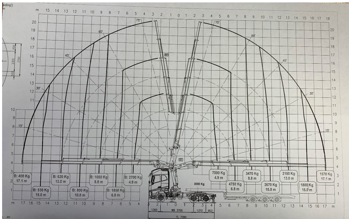
Merk: Volvo Kraantype: HMF 4220K6
